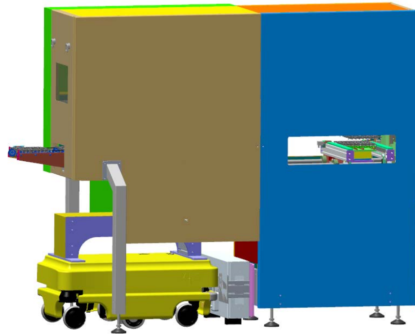
Asservimento automatico di una serie di robot per manipolazione telai di saldatura.
